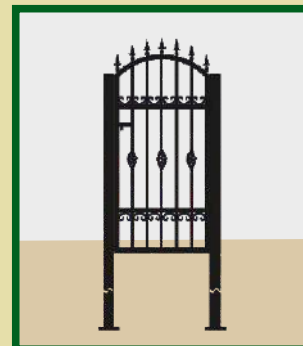
калитка с элементами ковки №3 1000x1750
