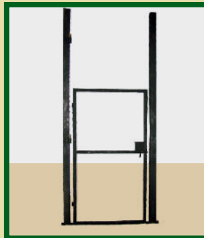
каркас калитки под профнастил 1000x1850
