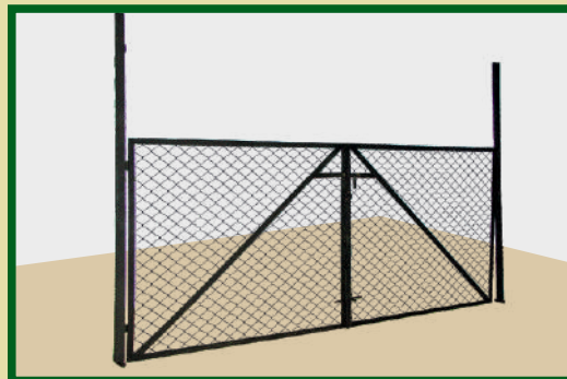
ворота с сеткой рабица 3500x1500
